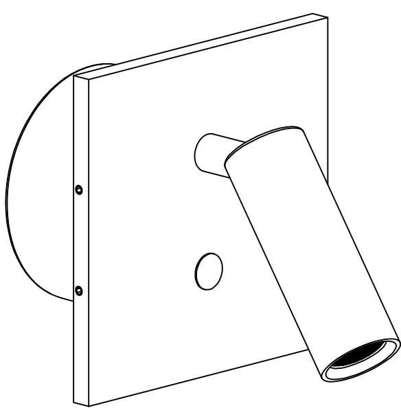
L110×W110×H105(mm)
