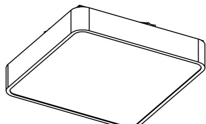
WYMIARY JĄŚ L400xW400xH82(mm) SMD-36W
