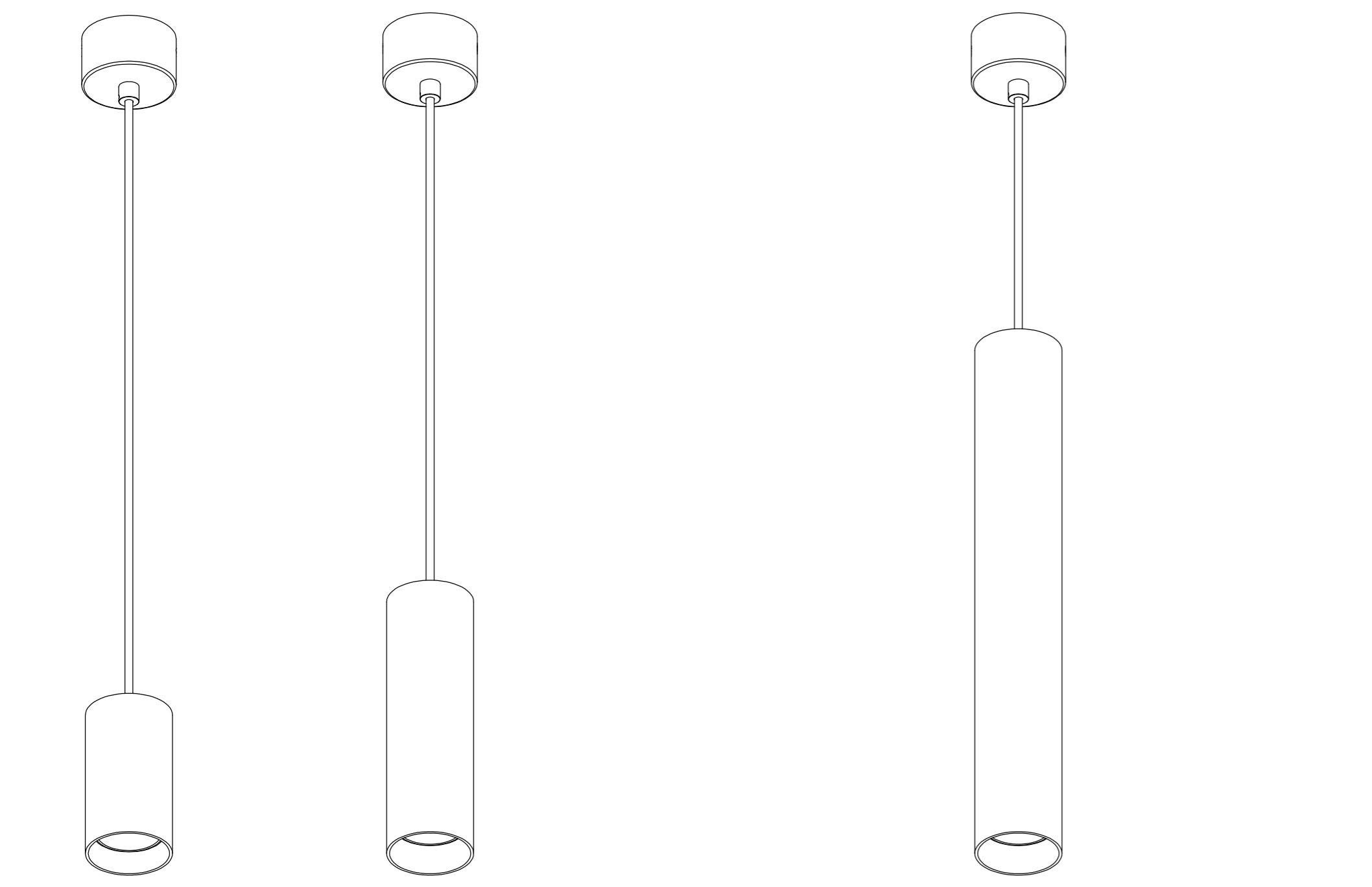
STALA/Z 010 M D65x110,H1200(mm) STALA/Z 010 L D65x200,H1200(mm) STALA/Z 010 XL D65x400,H1200(mm)
