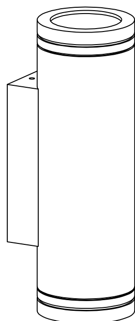
L74×W60×H190(mm) GU10
