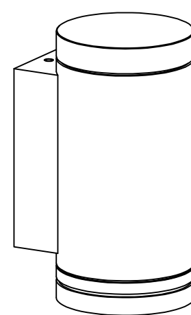
L74×W60×H125(mm) GU10
